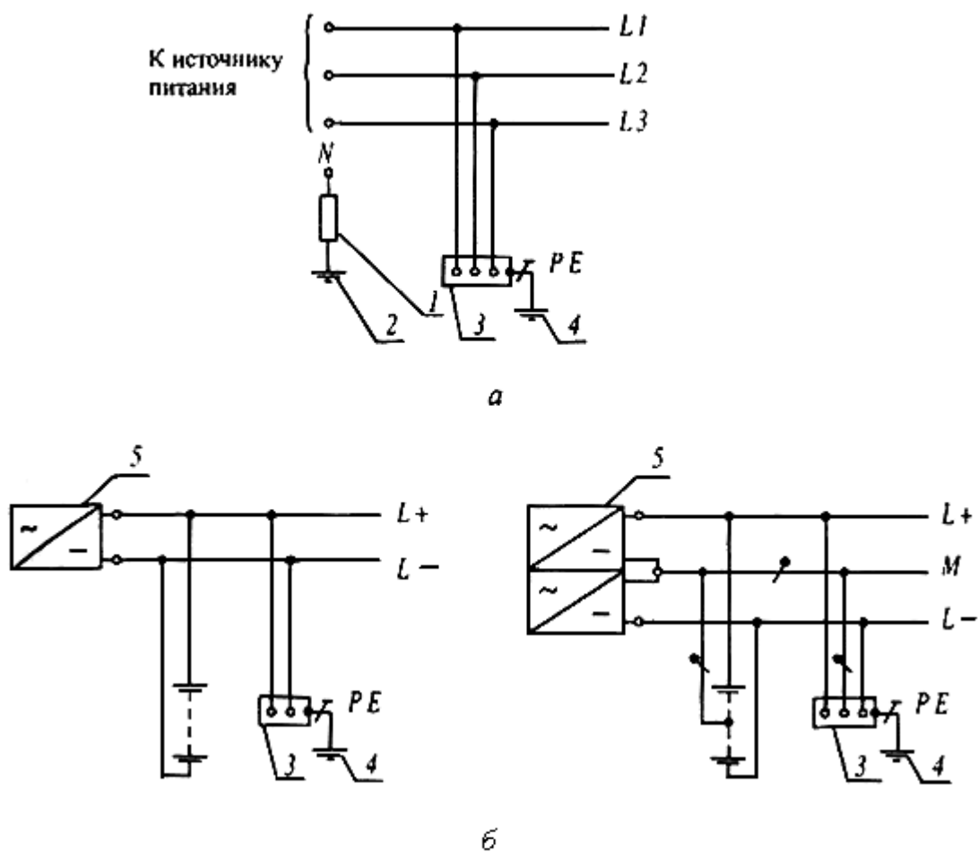
Рис.1.7.4. Система IT переменного ( a ) и постоянного ( b ) тока. Открытые проводящие части электроустановки заземлены. Нейтраль источника питания изолирована от земли или заземлена через большое сопротивление:
