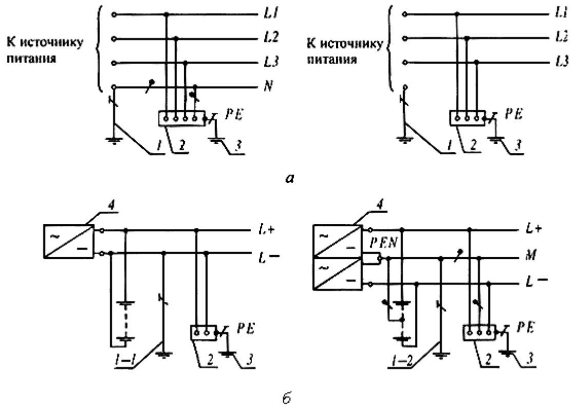
Рис.1.7.5. Система TT переменного ( a ) и постоянного ( b ) тока. Открытые проводящие части электроустановки заземлены при помощи заземления, электрически независимого от заземлителя нейтрали: I - заземлитель нейтрали источника переменного тока; I-1 - заземлитель вывода источника постоянного тока; I-2 - заземлитель средней точки источника постоянного тока; 2 - открытые проводящие части; 3 - заземлитель открытых проводящих частей электроустановки; 4 - источник питания
